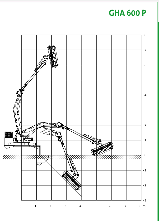
Reichweitendiagramm GHA 600 P
