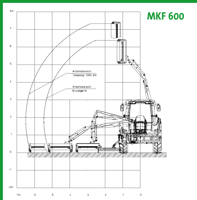
Reichweitendiagramm des MKF 600 am Steyr CVT
