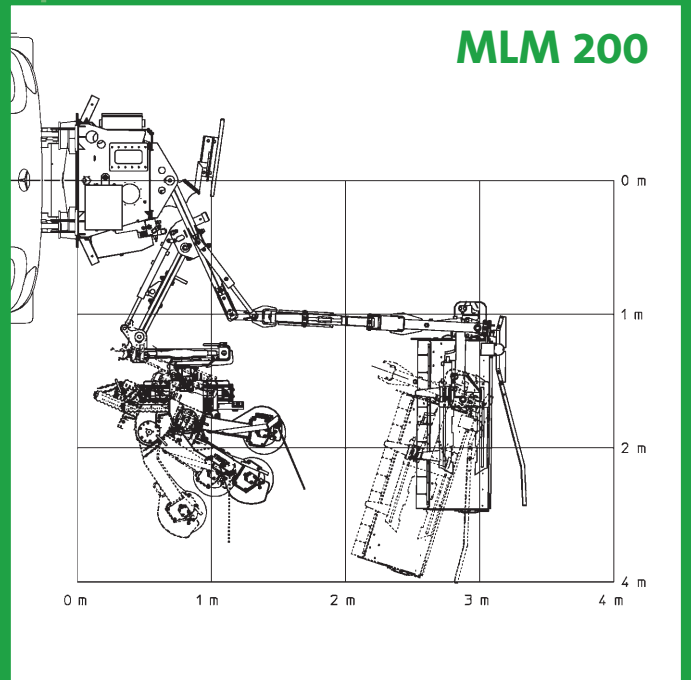
Reichweitendiagramm MLM 200
