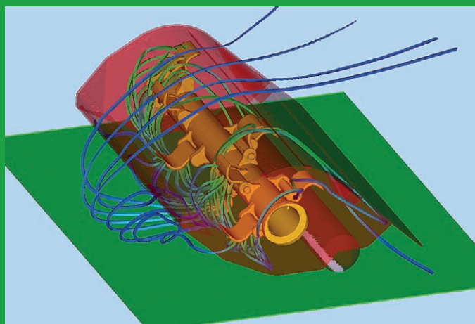
Strömungsoptimierung durch moderne Computersimulationen
